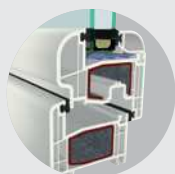
Sistema con anta semi- complanare a 5 camere
